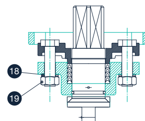
A-A VIEW
